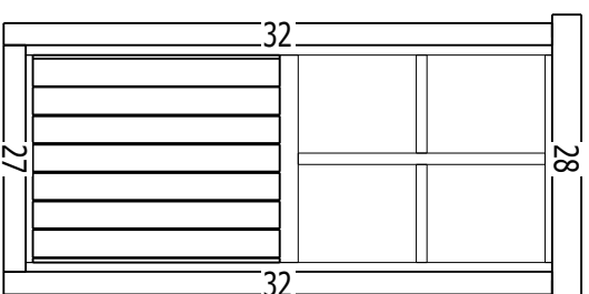
DOOR 850X1920
