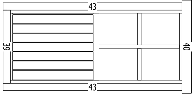
DOOR 850X1920
