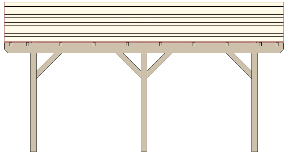
Right Elevation
