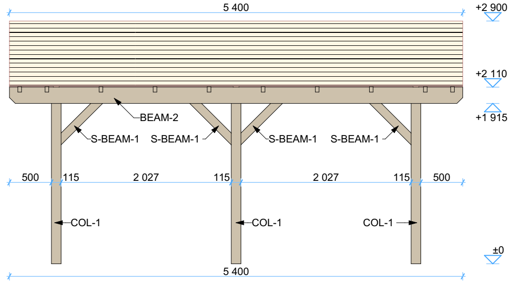
Right Elevation
